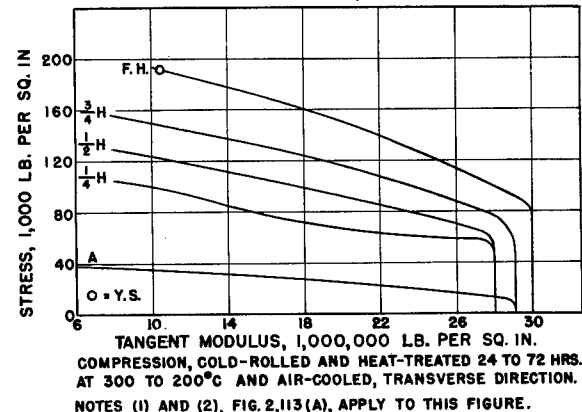
FIGURE No. 2.113 (d)
